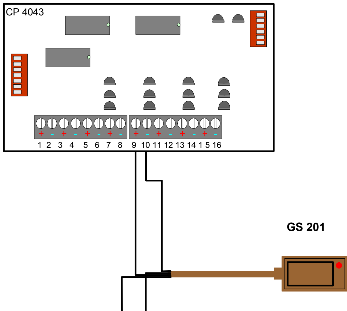
Abbildung 27: Anschaltung Glasbruchmelder GS 200 an CD 15004
