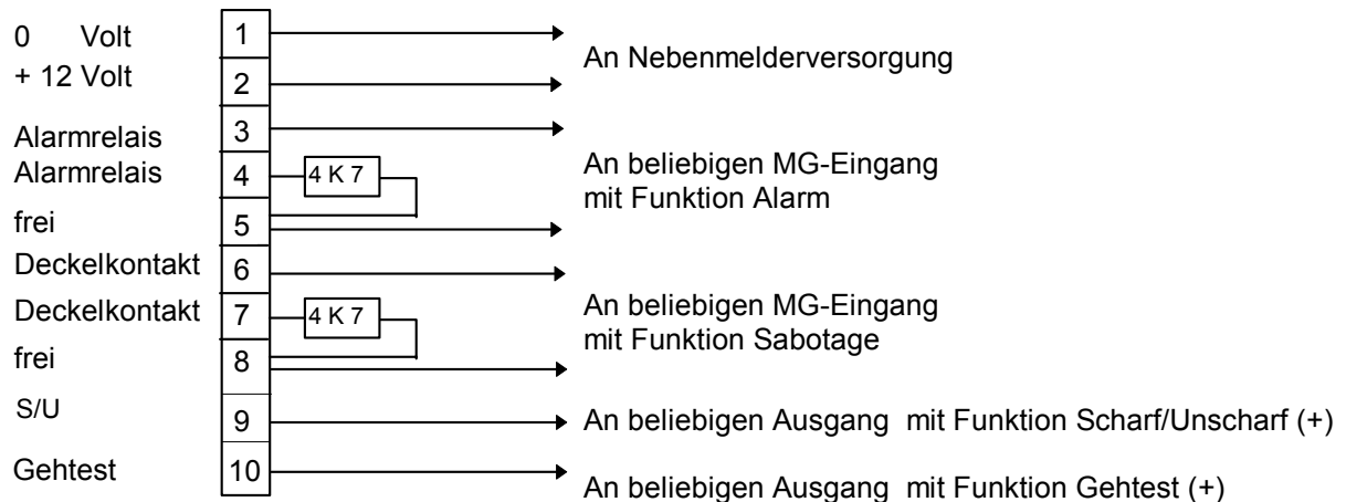
Abbildung 30: Bewegungsmelder mit Speicher
