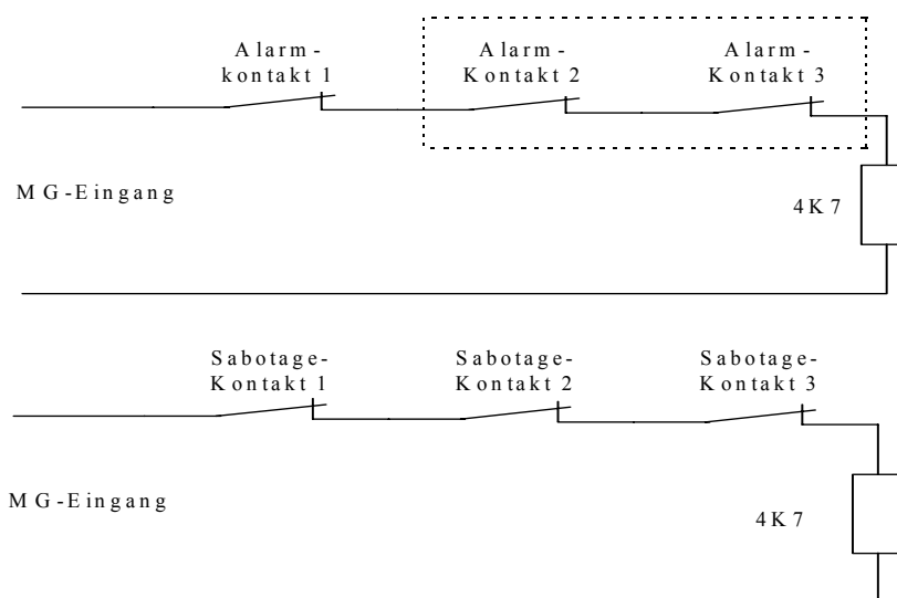
Abbildung 1: Getrennte Alarm- und Sabotage-MG
