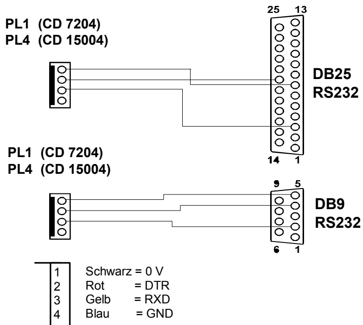
Abbildung 35: Druckeranschluß
