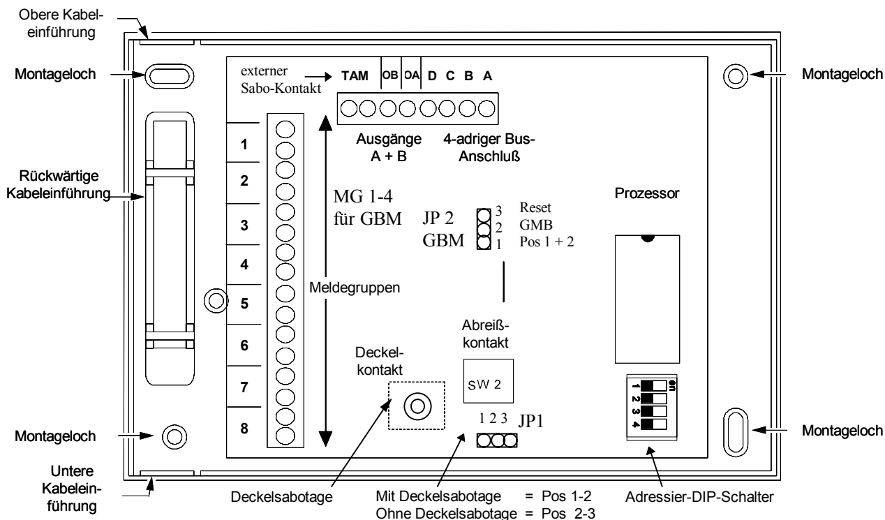
Abbildung 13: CD9041 Meldegruppen-Erweiterung
