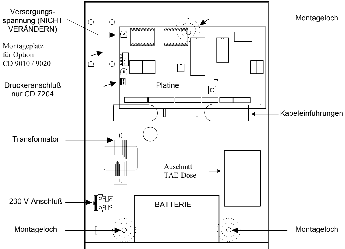
Abbildung 4: Das Gehäuse der CD 3404 / CD7204
