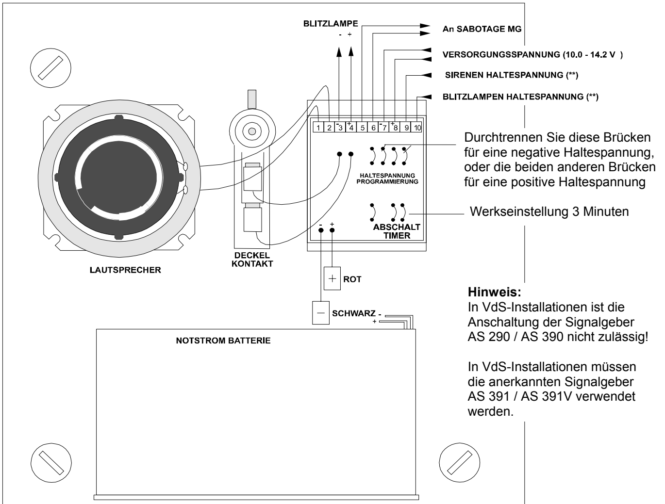
Abbildung 37: Außensirene AS 290 / 390
