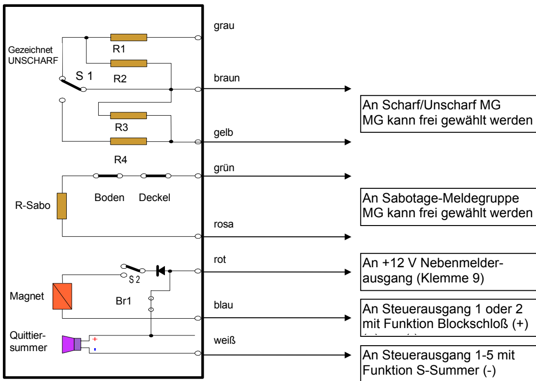
Abbildung 19: Anschaltung Blockschloß CD 225 DB/PZ an CD 3404 und CD 7204
