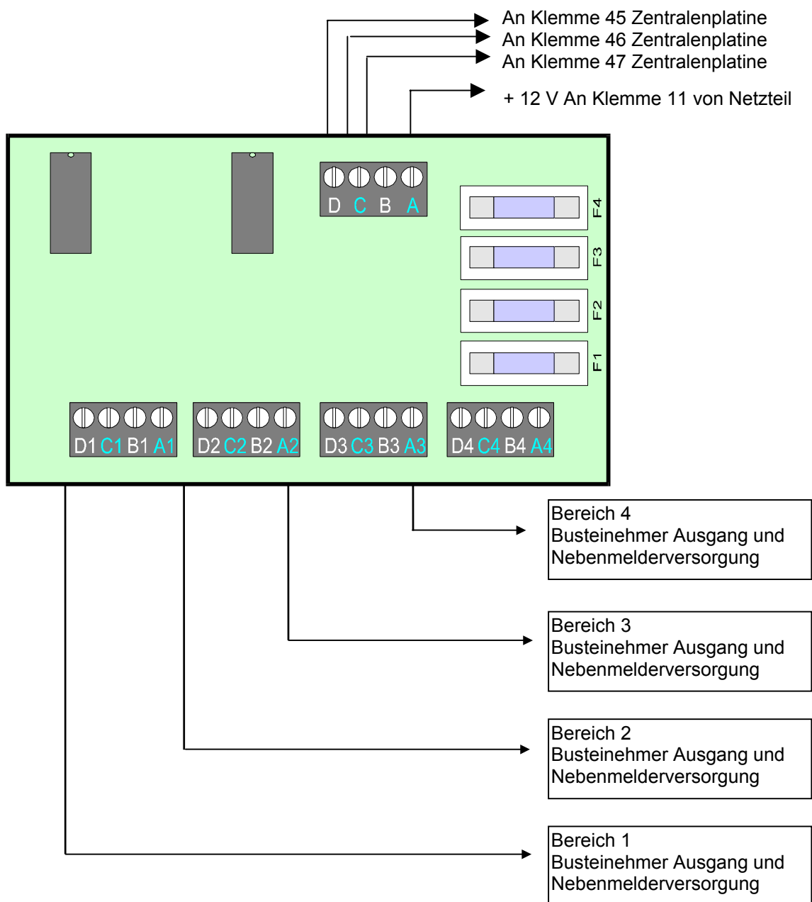
Abbildung 24: Anschaltung CD 9010 an CD 15004
