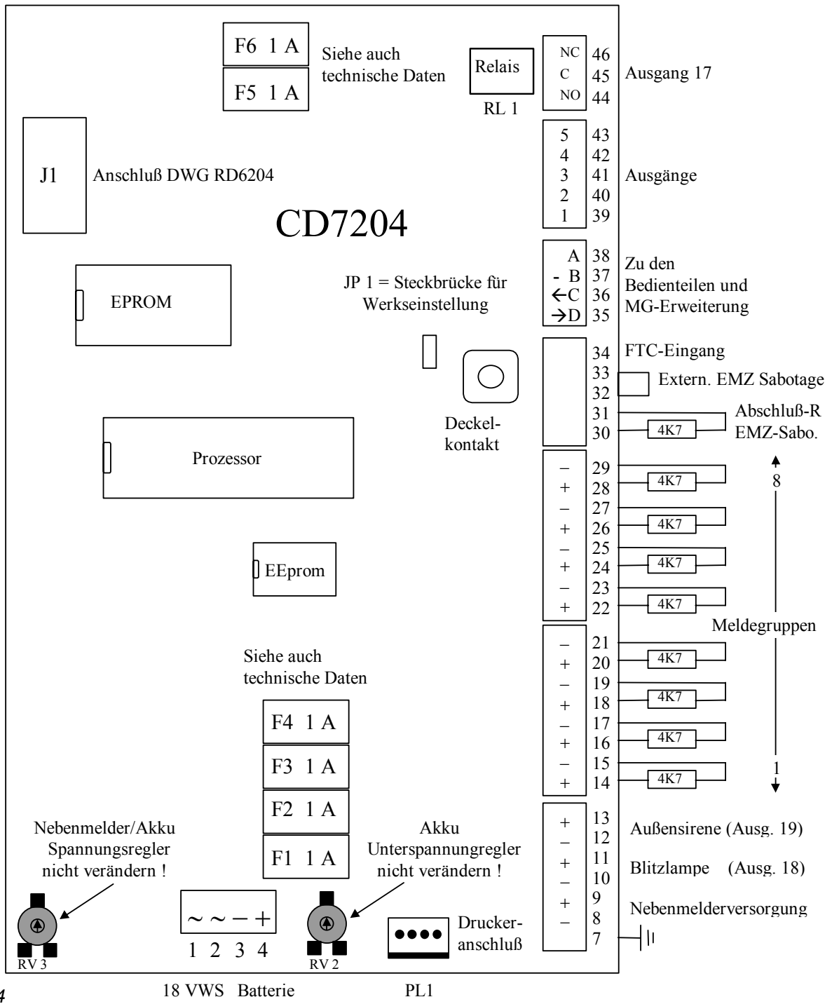
Abbildung 6: Alarmzentrale
