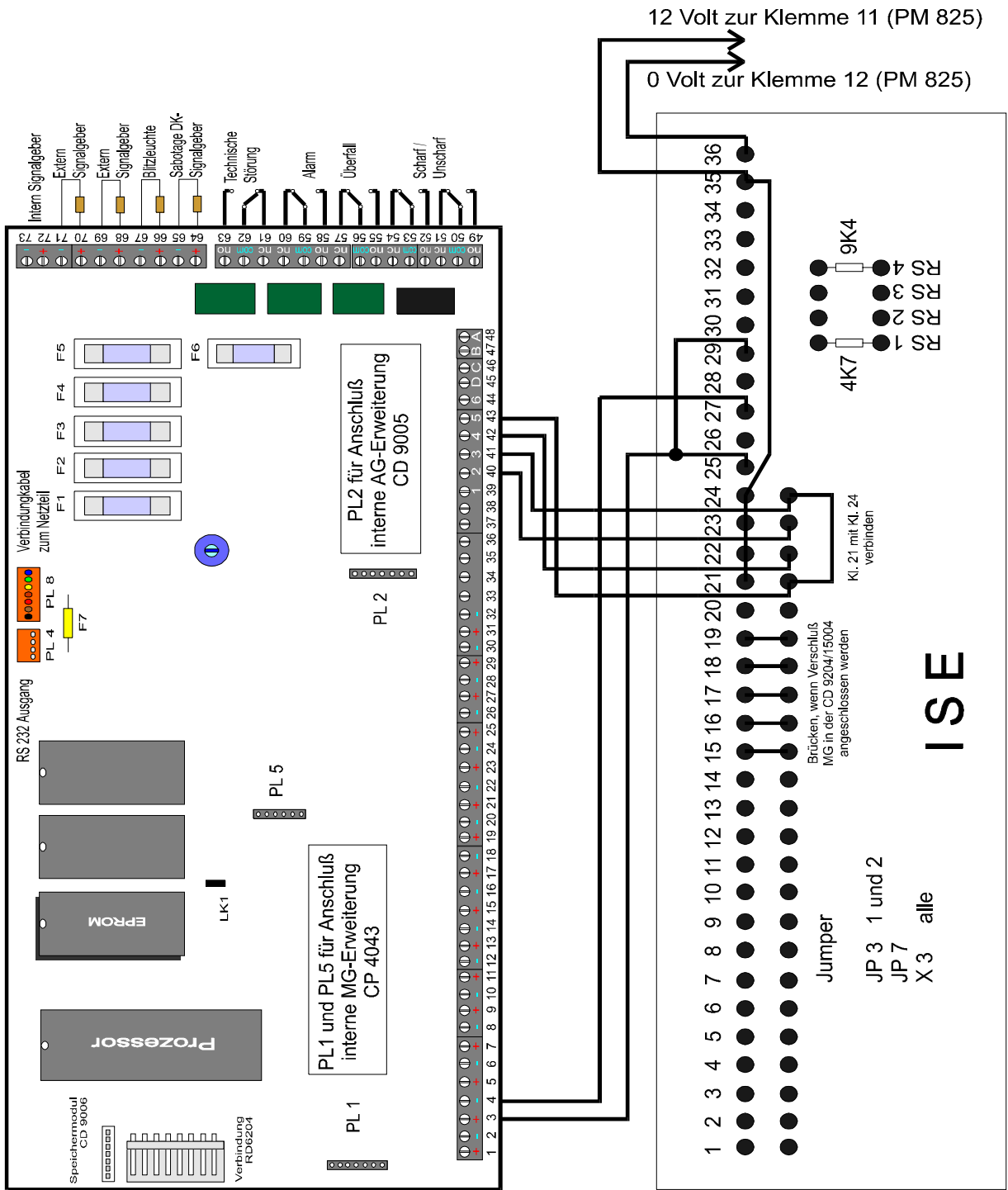
Abbildung 23: Anschaltung ISE an CD 15004
