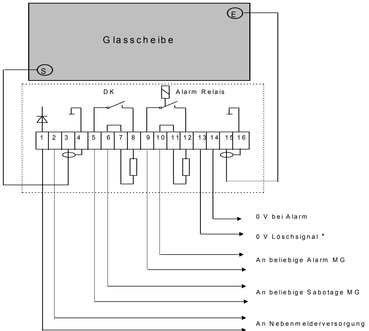
Abbildung 28: Anschaltung MAGS an CD 15004
