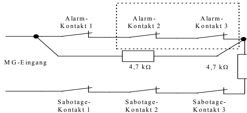
Abbildung 2: Gemeinsamer Anschluß der Alarm & Sabotage-MG
