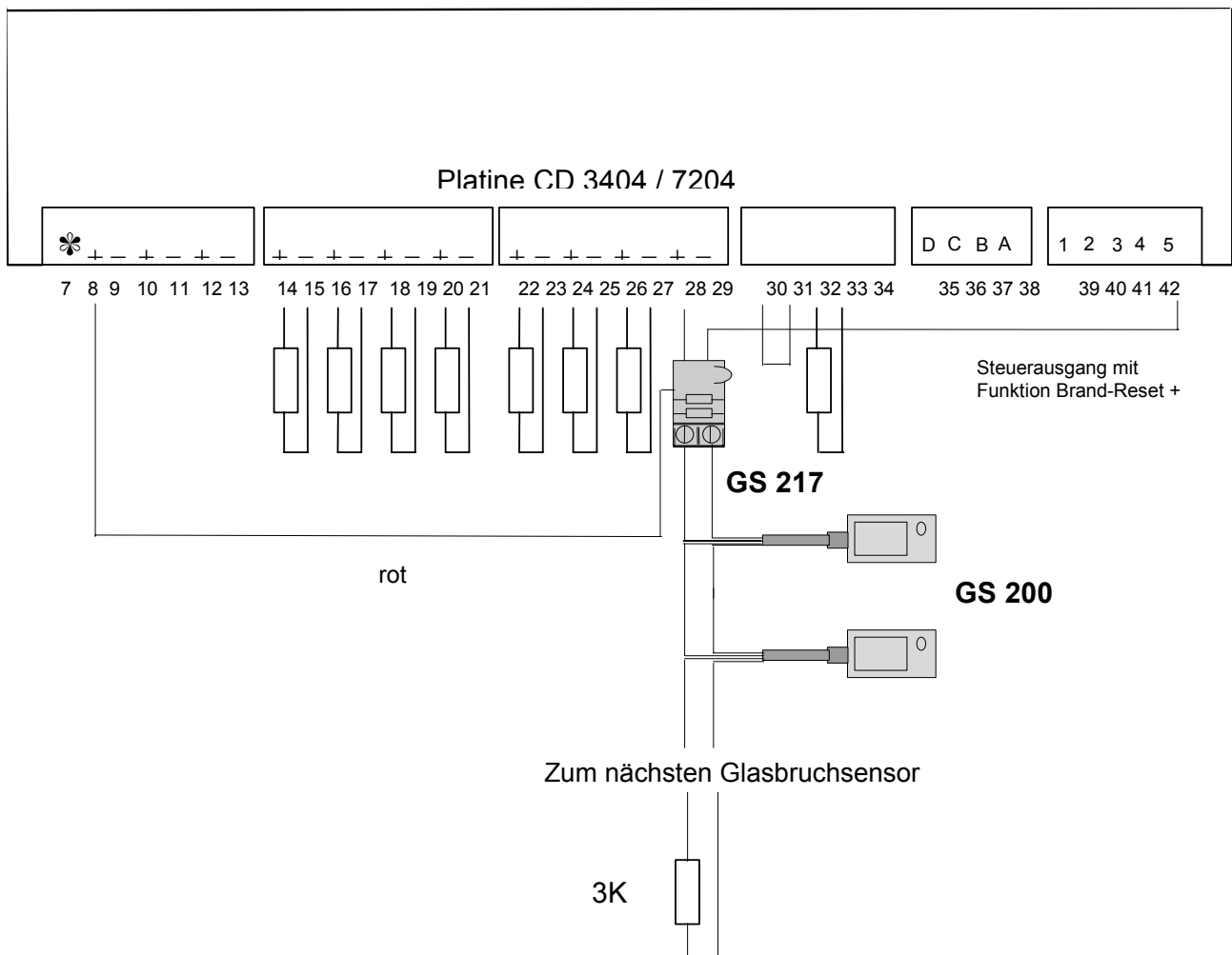
Abbildung 26: Anschaltung Glasbruchmelder GS 200 an CD 3404 und CD 7204
