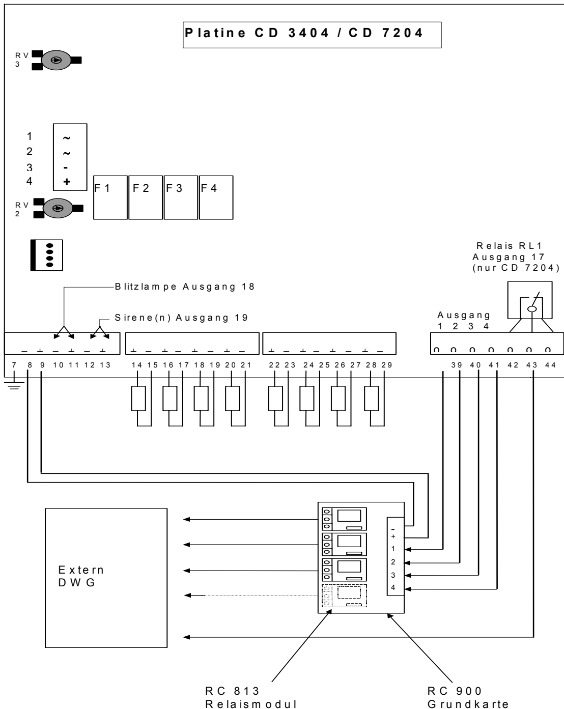
Abbildung 17: Anschaltung Extern Wählgerät an CD 3404 und CD 7204
