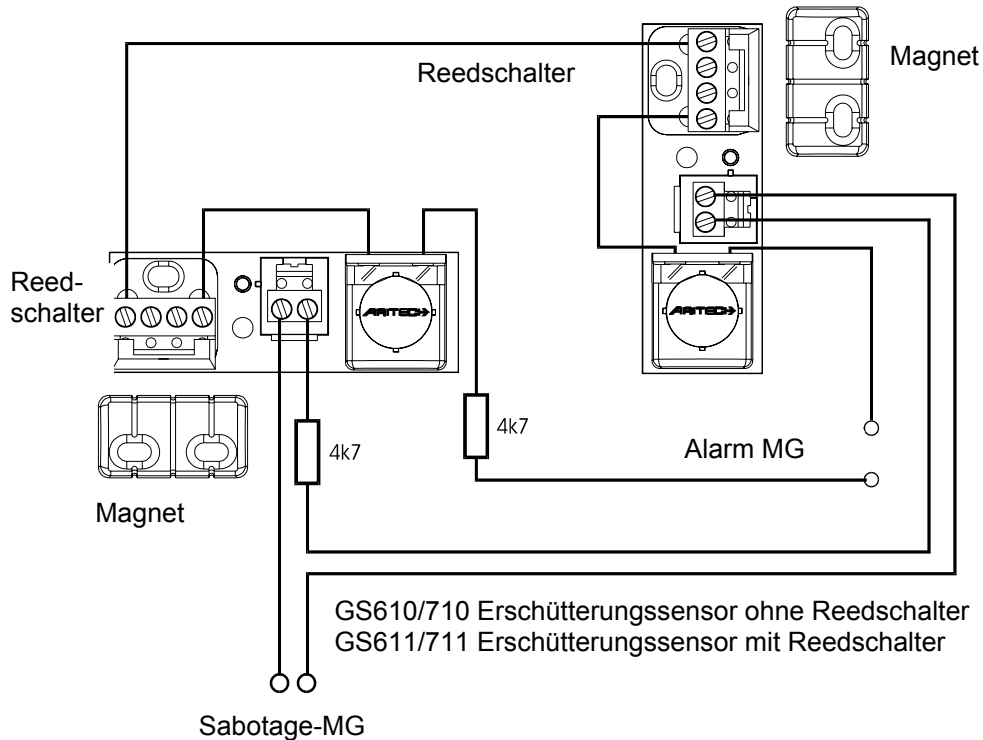
Abbildung 34: Anschluß eines GS710/711 mit kombinierten Alarm- & Sabotage-MG
