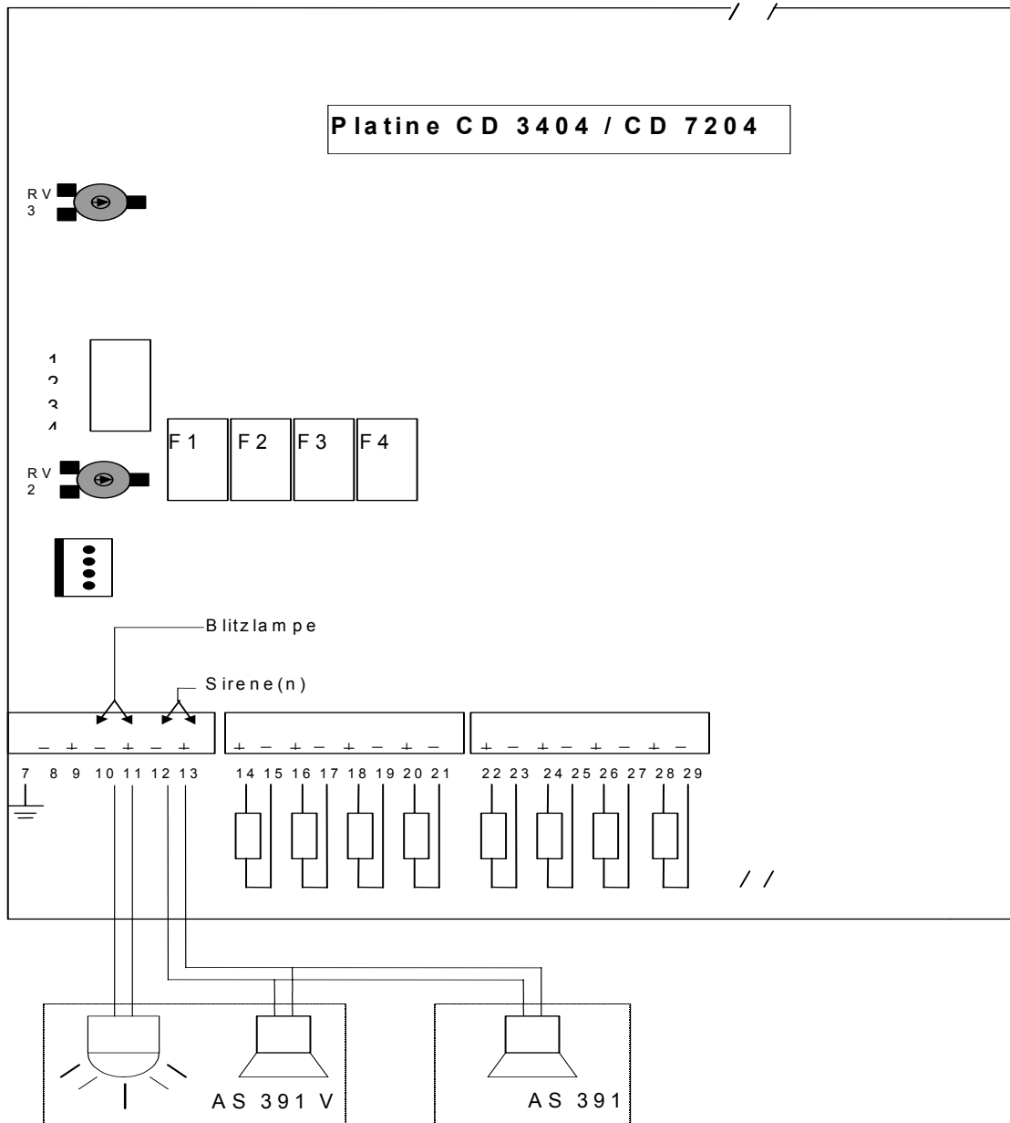
Abbildung 16: Anschaltung Externe Signalgeber an CD 3404 und CD 7204
