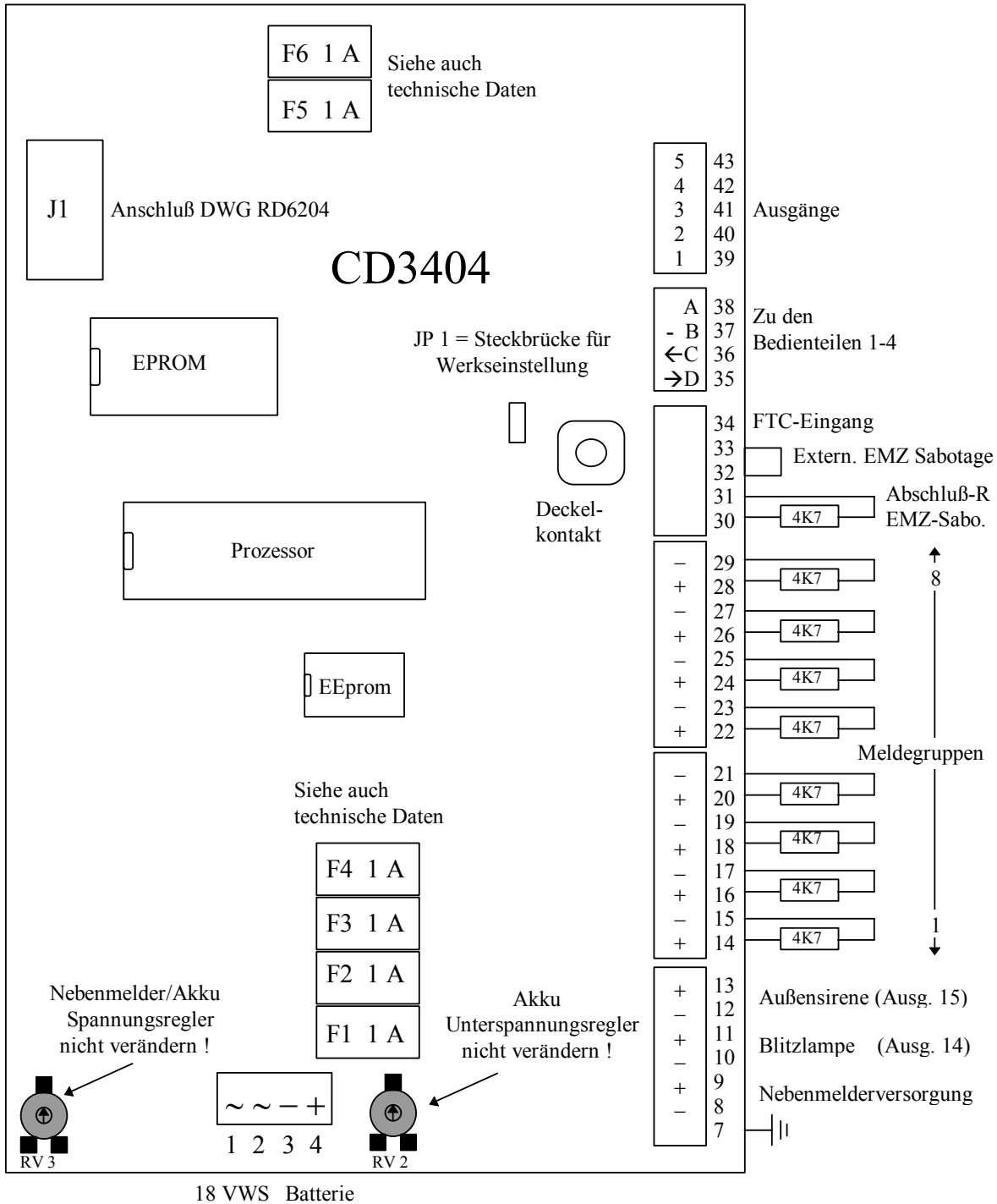
Abbildung 5: Alarmzentrale CD3404
