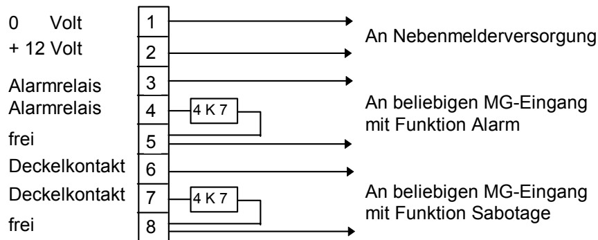
Abbildung 29: Bewegungsmelder ohne Speicher
